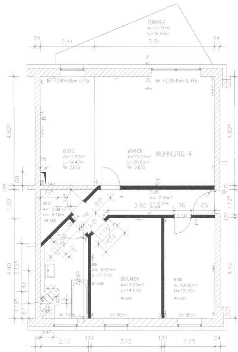
WE4 Kornblumenweg 3; M 1:100
